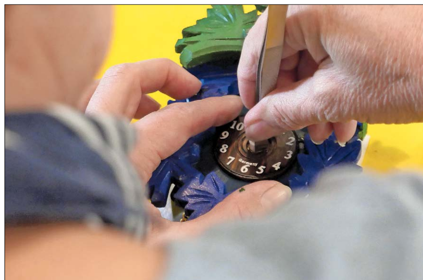
▲ Zum Schluss werden das Zifferblatt auf die Vorderseite geklebt und die beiden Zeiger für die Stunden und für die Minuten eingesetzt.
