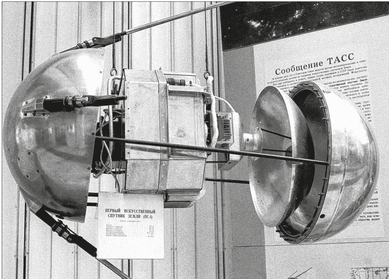
▲ Ein Modell von Sputnik 1 zeigt das Innenleben des Satelliten: Er trug zwei Funksender für codierte Kurzwellensignale, in denen Innendruck und -temperatur verschlüsselt waren. Zudem enthielt er drei Silber-Zink-Akkus und ein Wärmeregulationssystem, das mit Ventilatoren und Sensoren für Innen- und Außentemperatur ausgestattet war. Fotos: imago (3)
